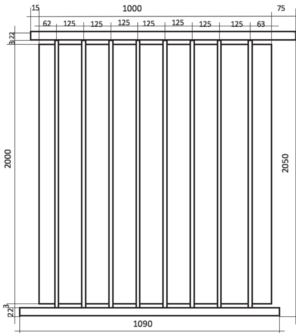
Схема абсорбера з розмірами
