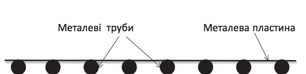
Поглинаюча панель (абсорбер) в розрізі
