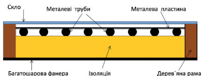
Розріз колектора
